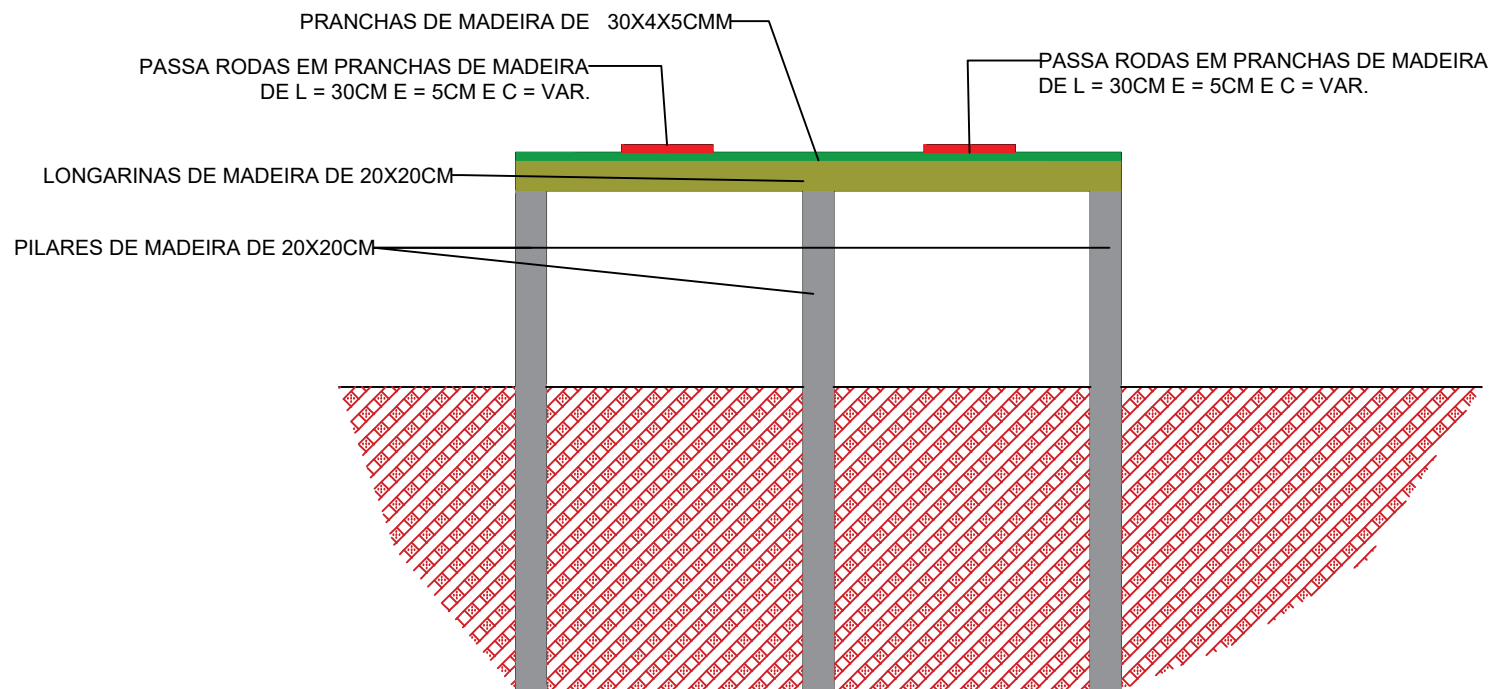
CORTE AA PONTE DE MADEIRA COM LARGURA = 4,00M E COMPRIMENTO VARIANDO DE 4 A 6,00M
