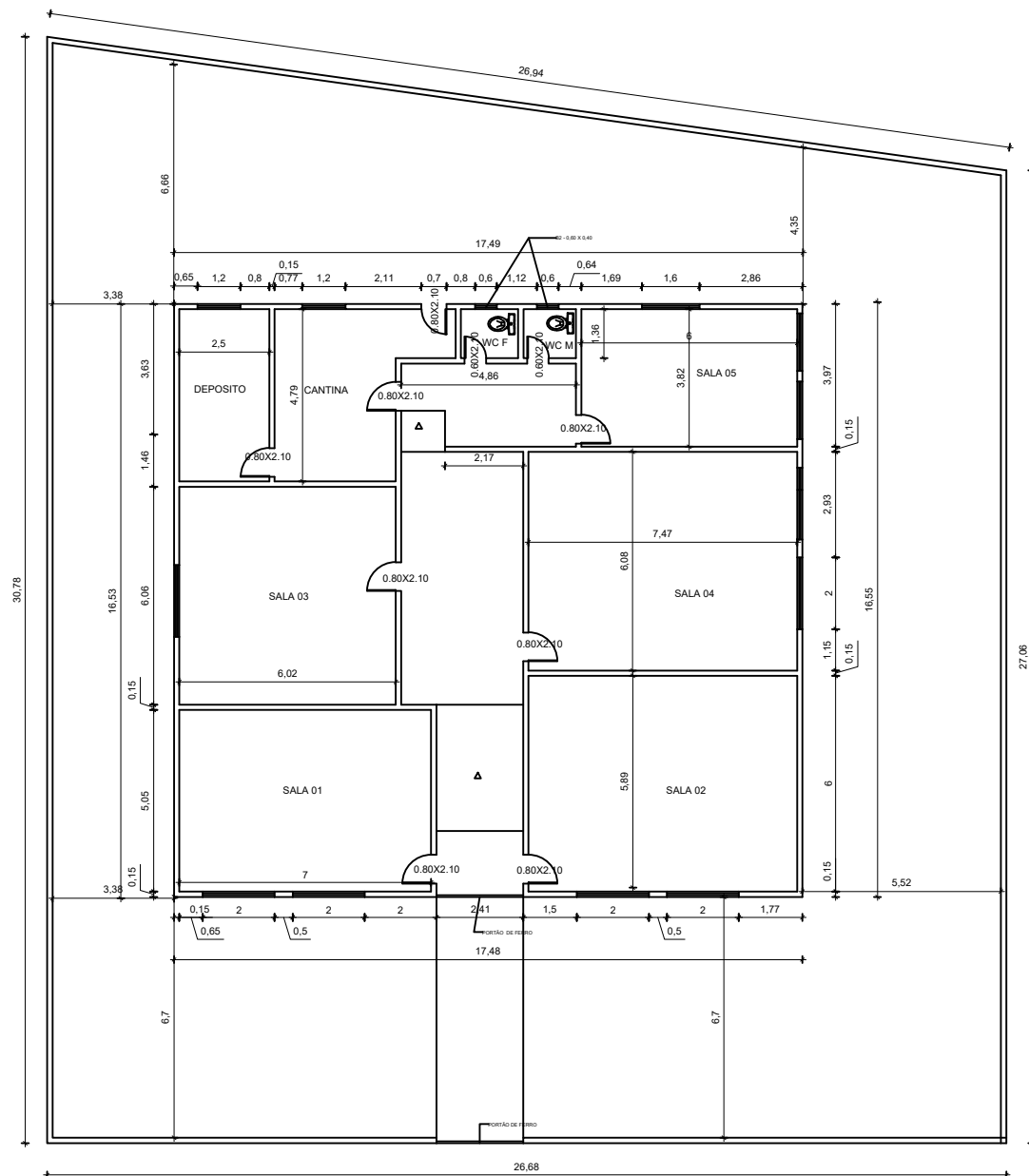
E.M ELISA MONTEIRO - BAIRRO MONTE CRISTO - SEDE PLANTA BAIXA
